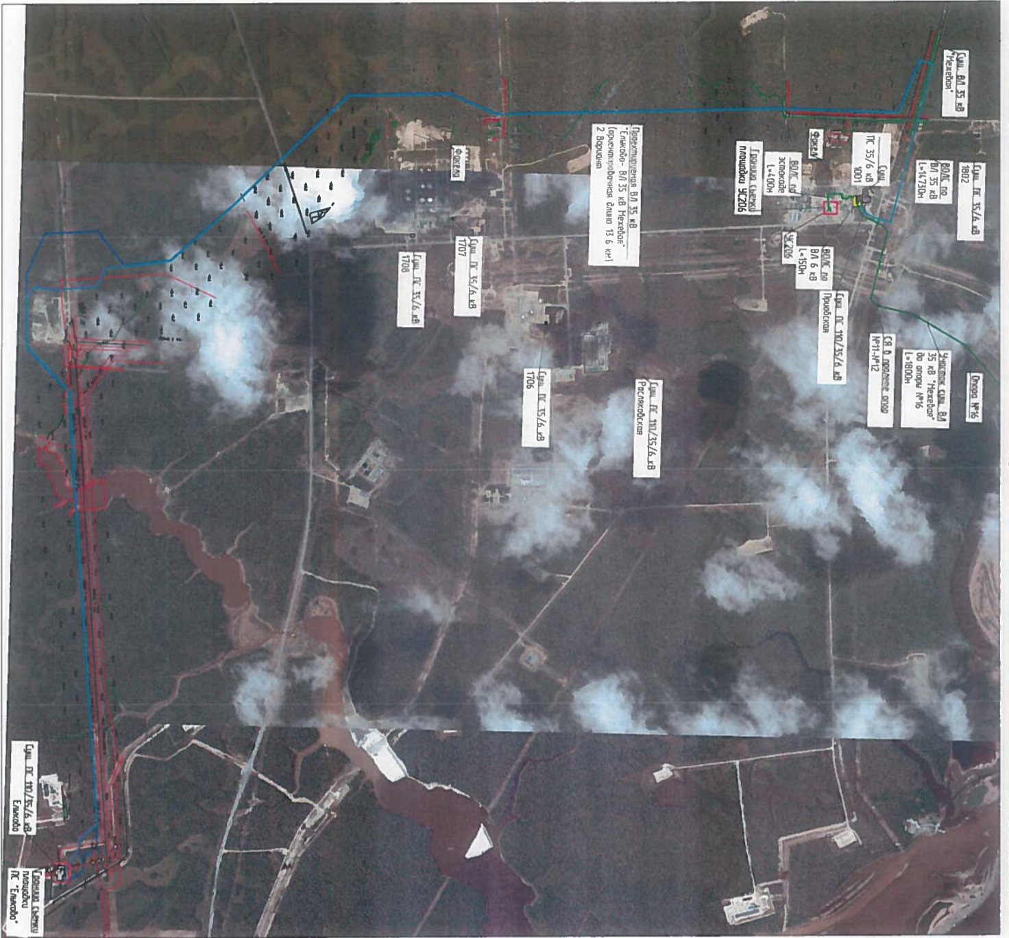
Предварительная схема площадок и трасс проектируемой ВЛ 35 кВ "Ельковд-ВЛ 35 кВ Межевод" (М 1:20000)
